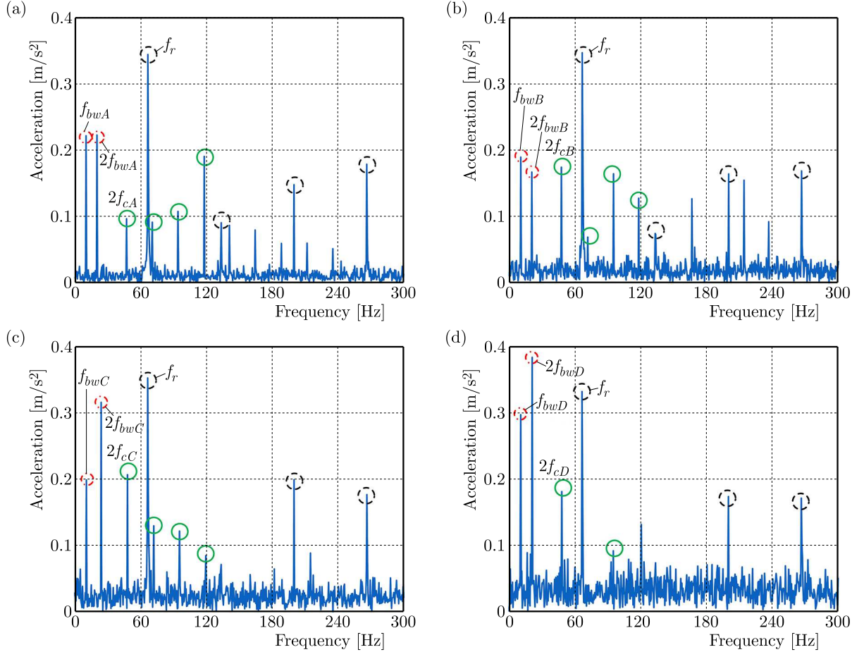
Fig. 9. Vibration spectrum of bearing dynamics model simulation: (a) A, (b) B, (c) C, (d) D
